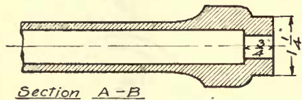
Section A-B
